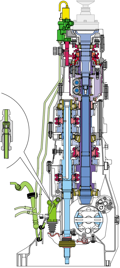
6-Gang-Schaltgetriebe 01E mit Nachschaltstufe
