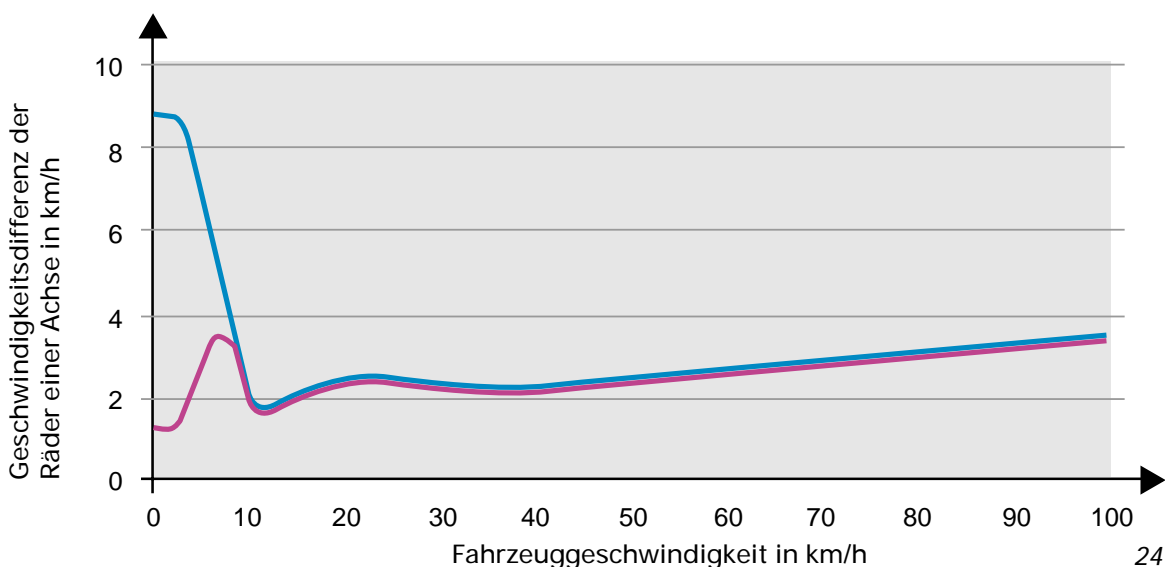
Vergleich der EDS-Anregelschwellen (Quersperre) bei Geradeausfahrt
