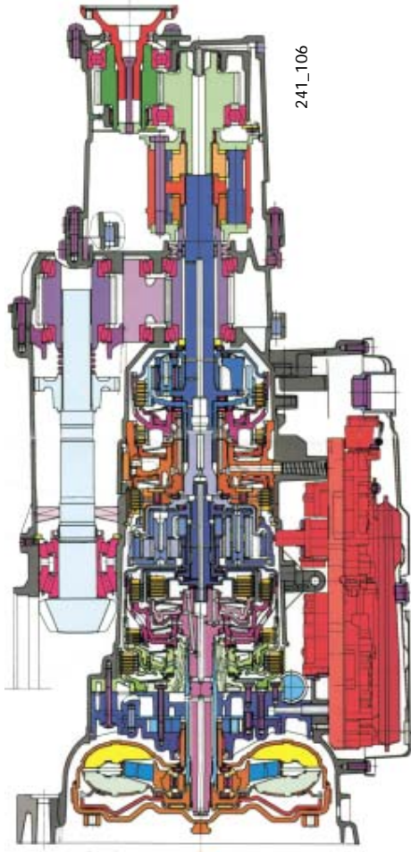
5-Gang-Automatikgetriebe 01V
