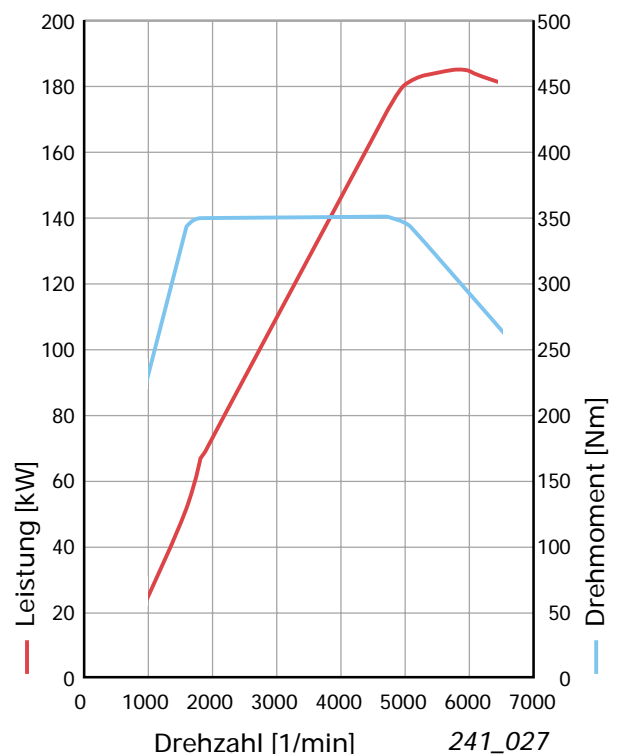
Motorkennbuchstabe: ARE
