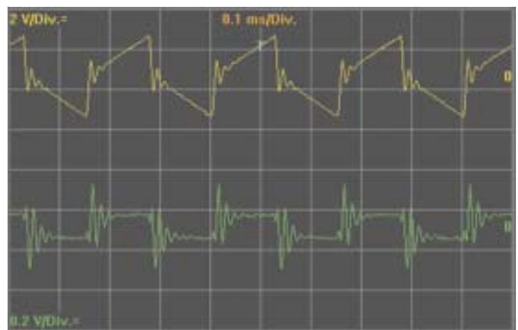
Signalbild Neutralstellung
